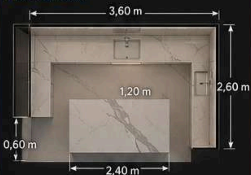
PLANTA BAIXA
